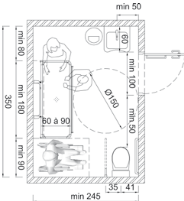
Salle d'hygiène disposant de toilettes, d'une aire de stationnement du fauteuil roulant et d'un second dégagement libre à l'extrémité de la table afin de permettre l'assistance d'une ou plusieurs personnes aidantes.
