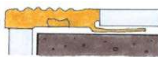
✓ Nez de marche antidérapant.
