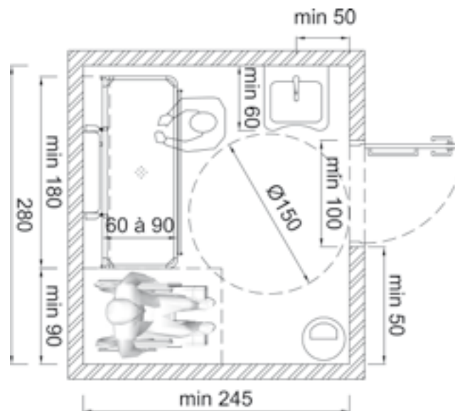
Salle d'hygiène disposant d'une aire de stationnement du fauteuil roulant afin de permettre l'assistance d'une personne aidante.
